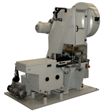
Disc-feed Press
